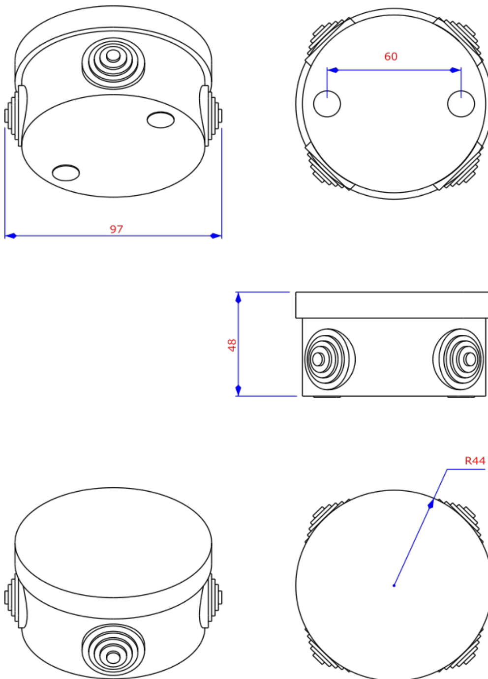
Рис. 2. Габаритные и установочные размеры ПР-3У IP55
