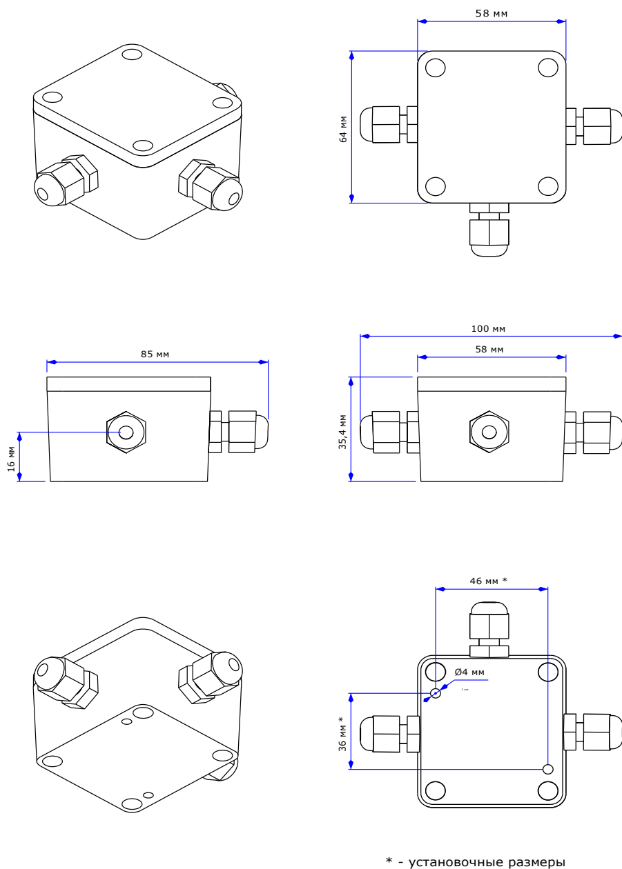
Рис. 2. Габаритные и установочные размеры ПР-3М IP65
