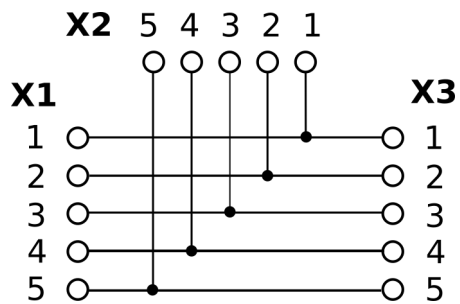
Рис. 1. Схема принципиальная ПР-3М
